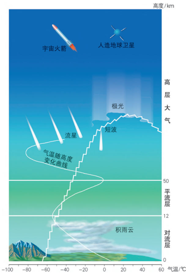
图2-1-2 大气的垂直分层示意
