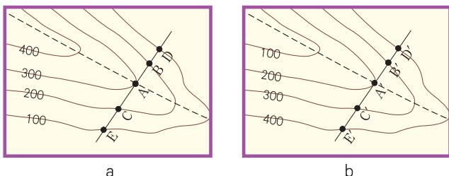
图3-5-4 山脊与山谷
