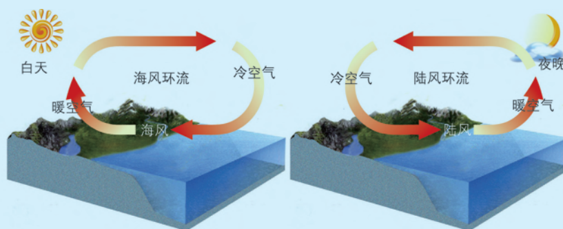
图2-1-10 海陆风形成示意
