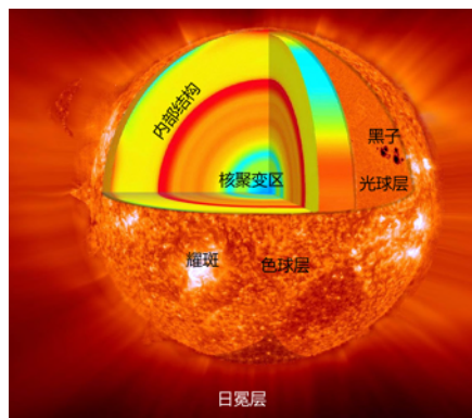
图1-1-13 太阳结构
