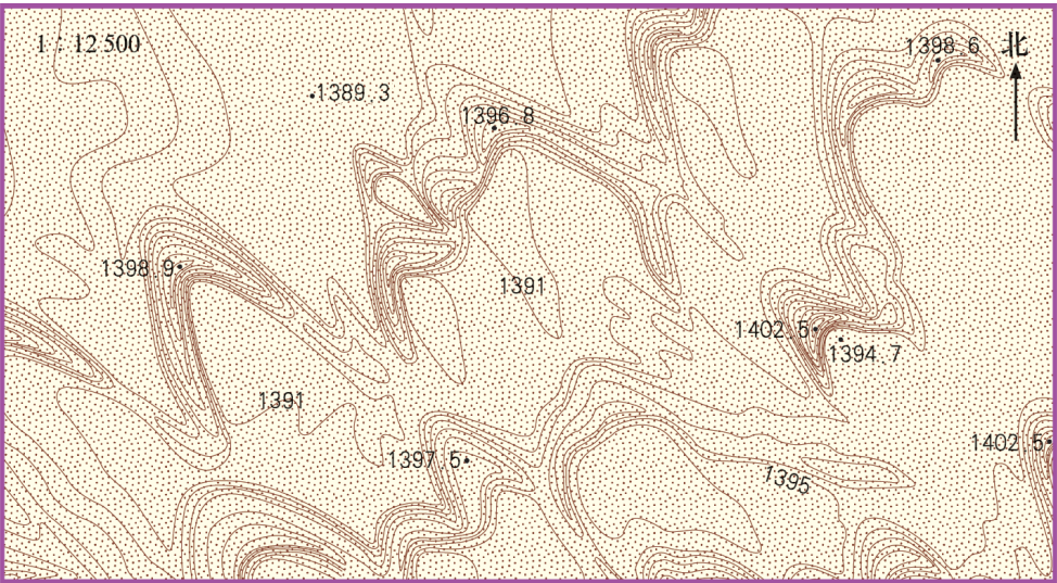
图3-5-7 沙丘等高线地形图
