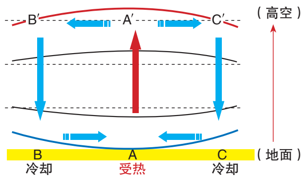
图2-1-9 冷热不均引起的热力环流示意
