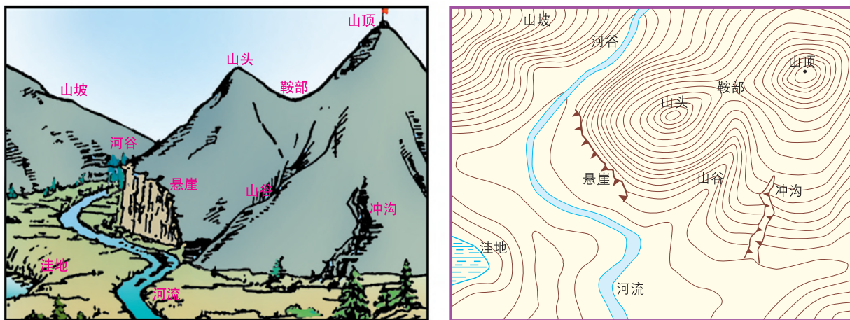
图3-5-6 地形景观与对应的等高线地形图
