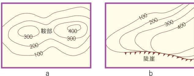
图3-5-5 鞍部与陡崖
