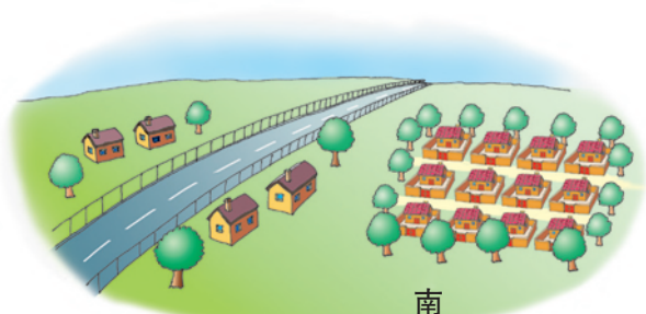
图1-4-7 根据房屋门窗朝向判别方向
