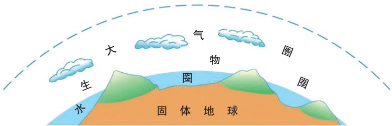
图1-3-4 地球外部圈层
