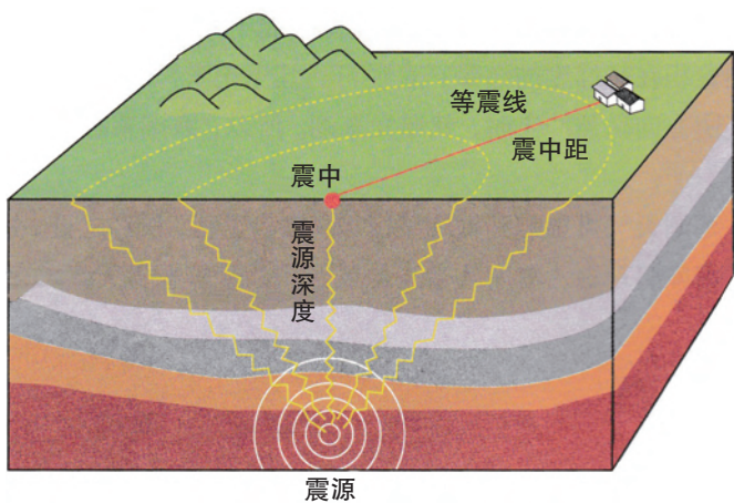
图4-1-4 震源、震中、震中距示意
