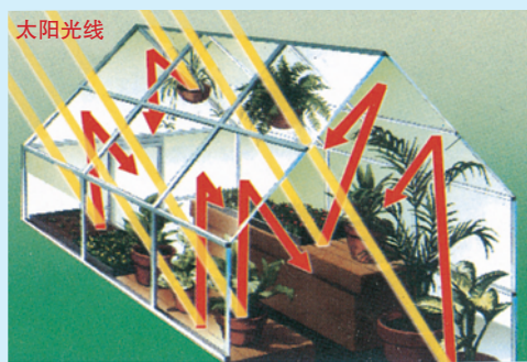
图2-1-7 玻璃暖房保温示意
