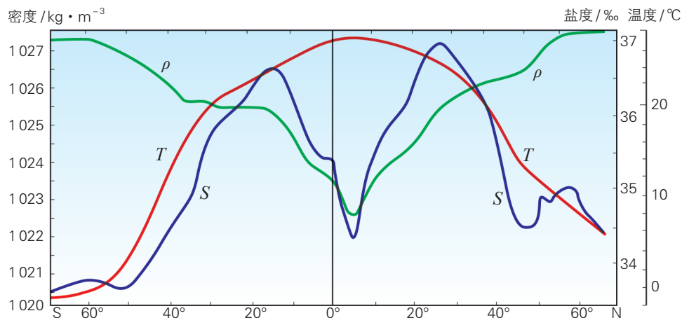
图2-2-7 8月大西洋表层海水温度、盐度、密度随纬度的变化
