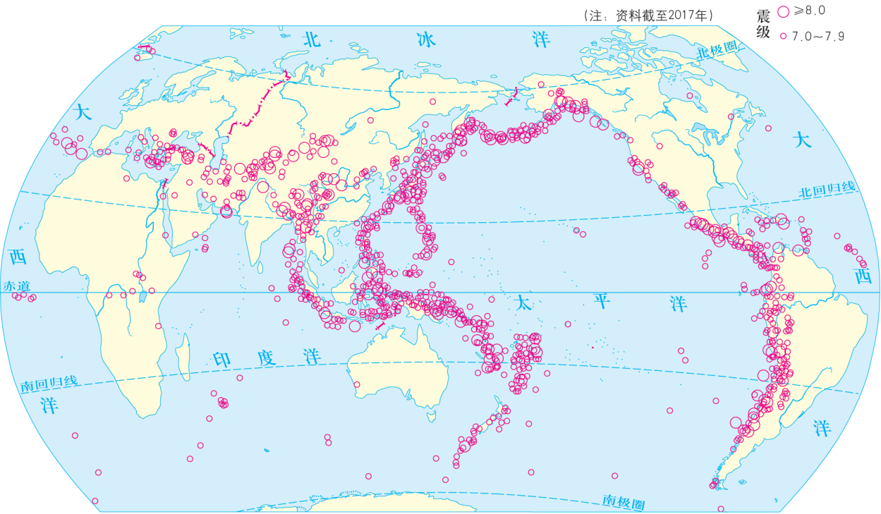
图4-1-5 世界7级以上大地震的震中分布
